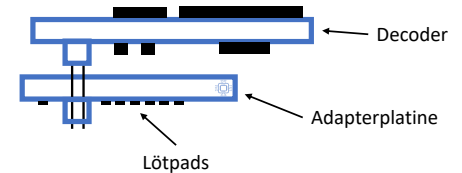
Abbildung 2: Montage des Decoders
